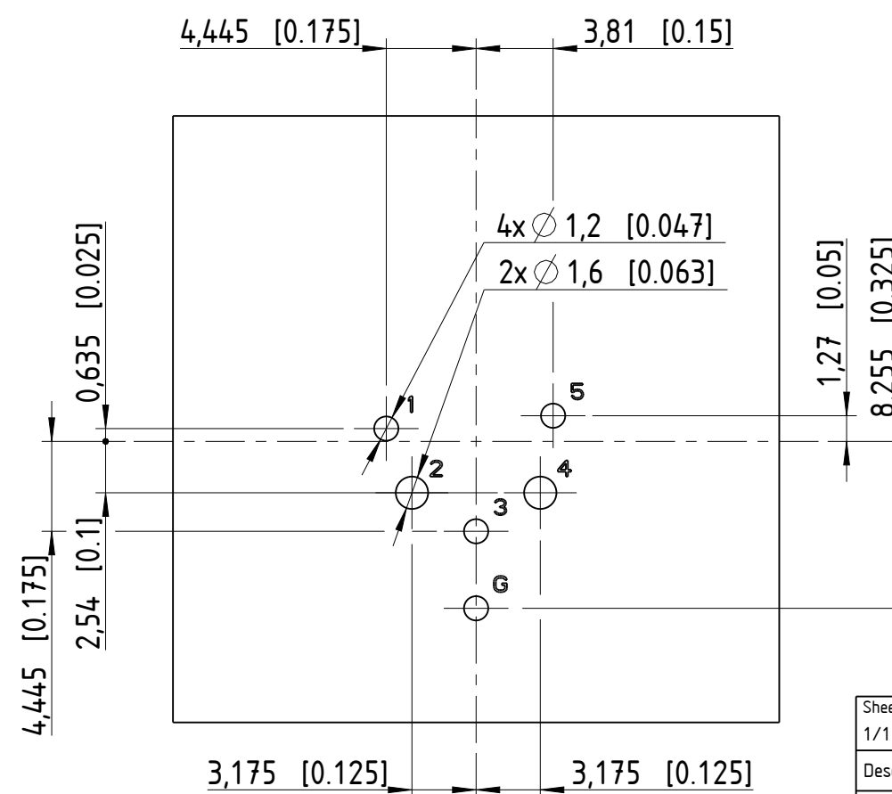
Printbohrplan (Bestückungsseite) PCB-Layer layout (component side)
