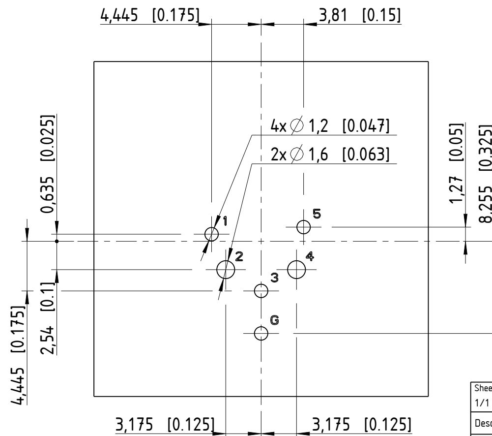
Print Bohrplan (Bestueckungsseite) Pcb-Layout (component side)
