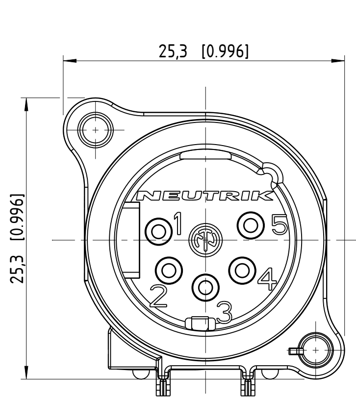
Frontplattenausschnitt (Rückseite) Panel cut ou (rear side)
