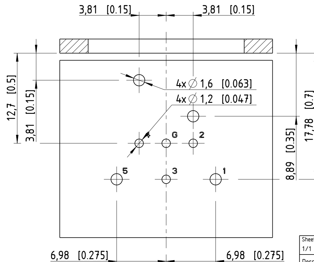
Print Bohrplan (Bestueckungsseite) Pcb-Layout (component side)
