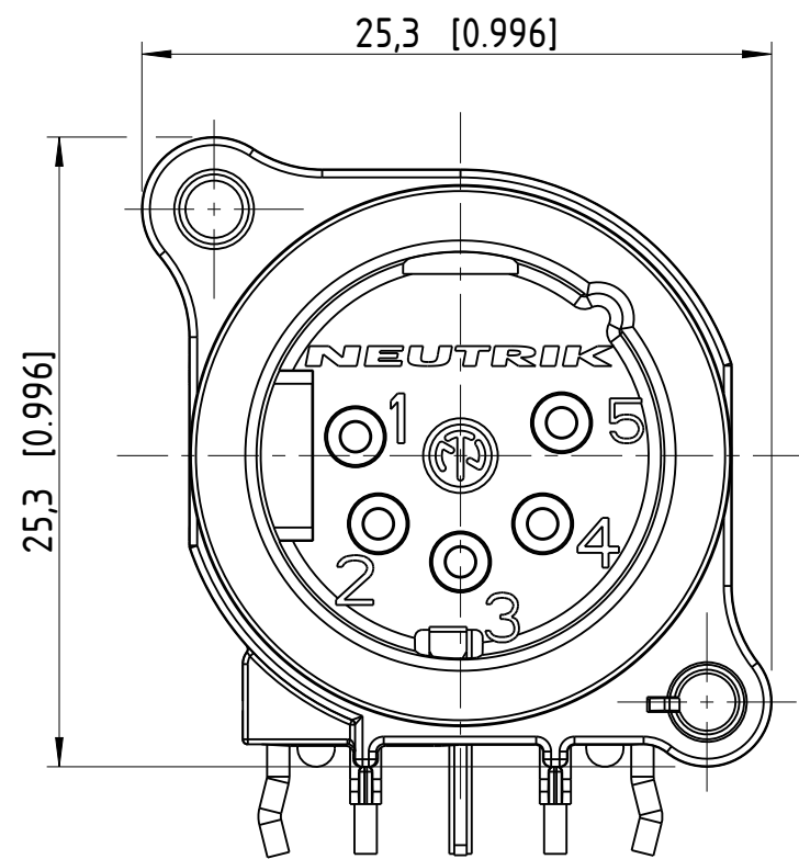
Frontplattenausschnitt (Rückseite) Panel cut ou (rear side)
