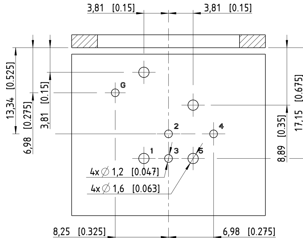
Print Bohrplan (Bestueckungsseite) Pcb-Layout (component side)
