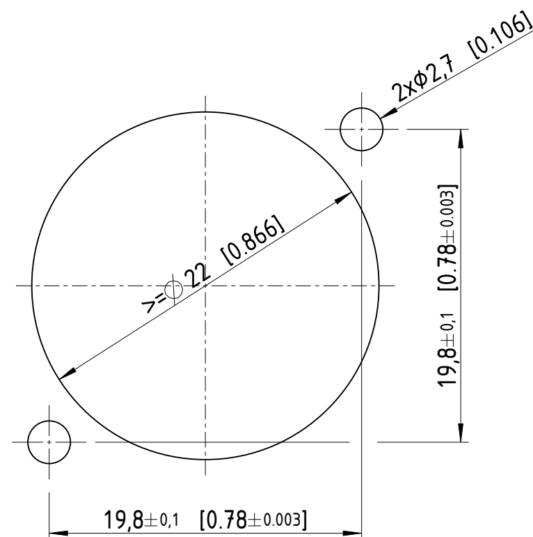
Frontplattenausschnitt (Rückseite)
