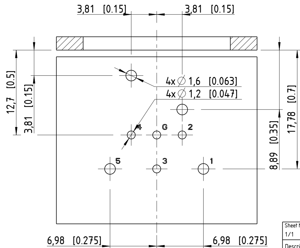
Print Bohrplan (Bestueckungsseite) Pcb-Layout (component side)
